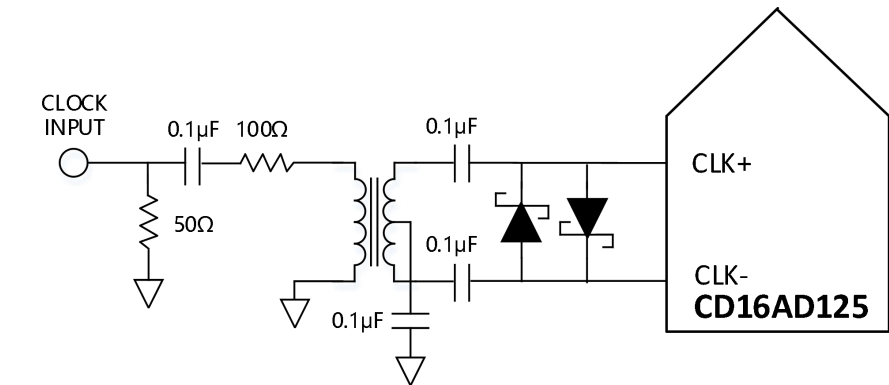
图 17.变压器配置的时钟输入
