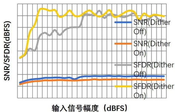
图 13. SFDR、SNR 与输入幅度的关系(fin=30.1MHz)
