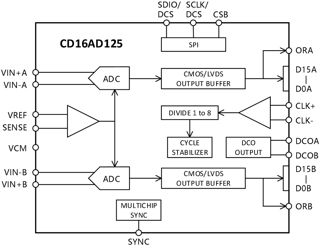
图 1. 功能框图
