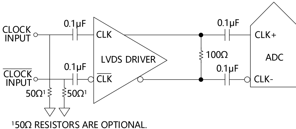
图 14. 时钟 LVDS 信号激励方案
