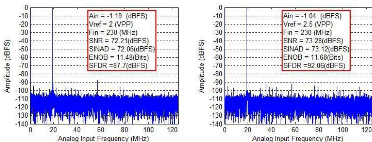
图 6. FFT 特性：模拟输入频率 230MHz、采样率 250MSPS
