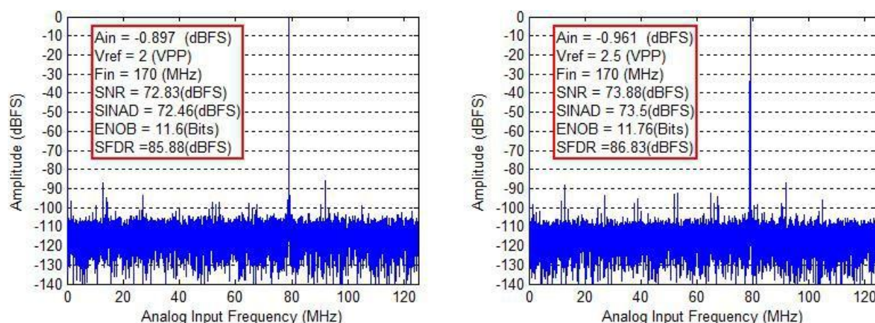
图 5. FFT 特性：模拟输入频率 170MHz、采样率 250MSP
