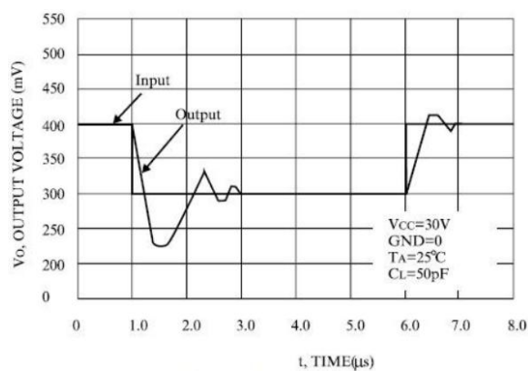
图 5.小信号电压跟随脉冲响应（非反向）
