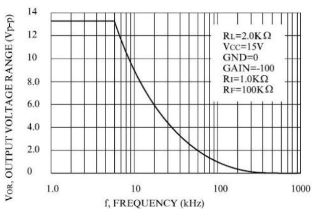
图 4.大信号频率响应
