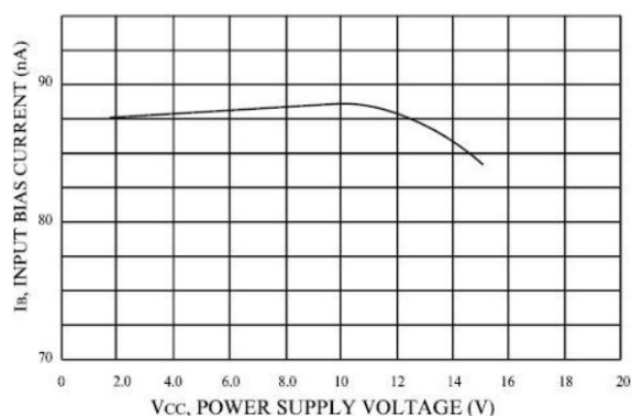
图 7.输入偏置电流 VS 电源电压
