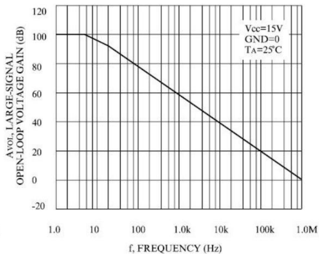
图 3.开环电压频率
