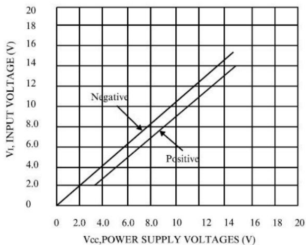
图 2.输入电压范围
