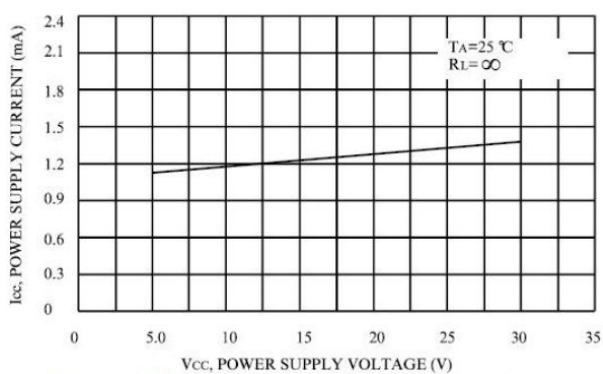
图 6.电源电压 VS 电源电流
