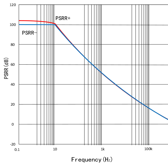
图 4. 电源电压抑制比 vs. 频率
