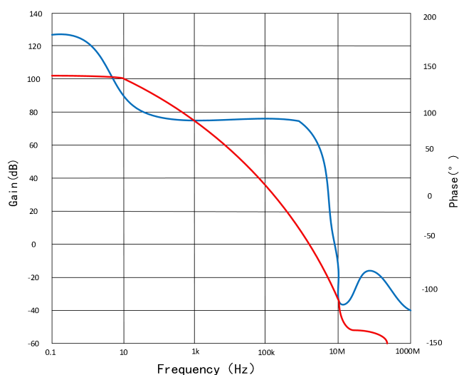
图 2. 开环增益 vs 相位
