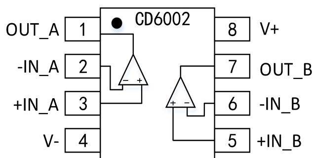
SOIC-8(SOP8) , MSOP-8
