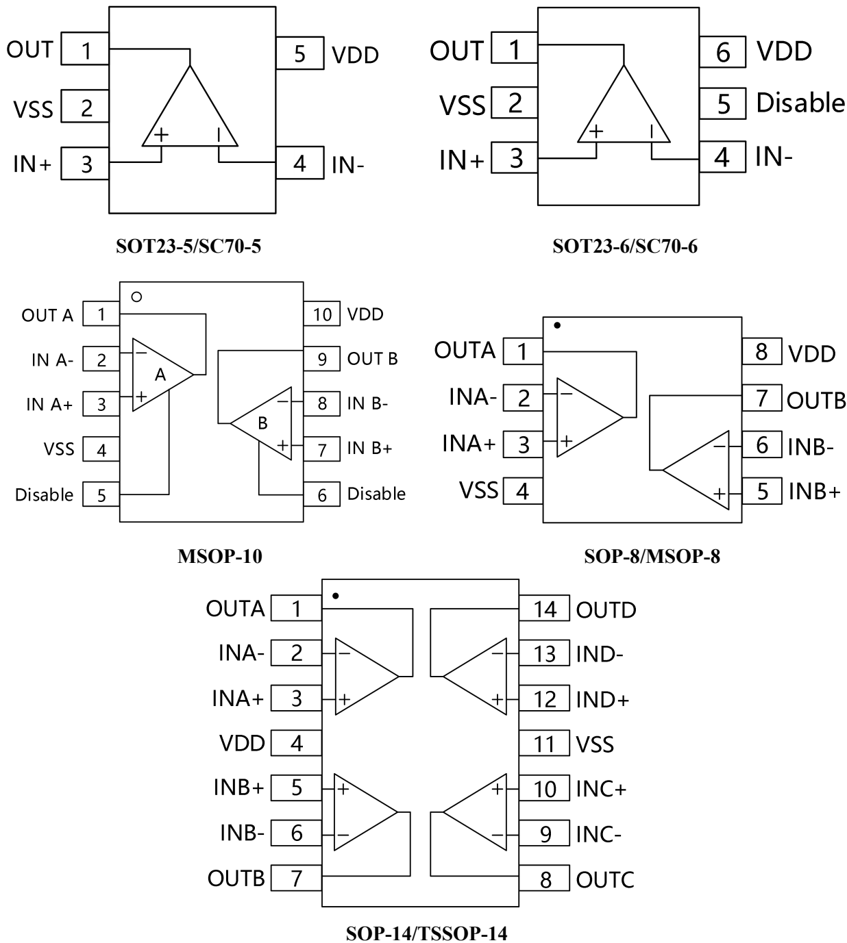
图 1. 引脚定义
