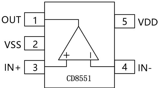
SOT23-5
