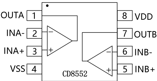
MSOP-8 / SOP-8/TSSOP8
