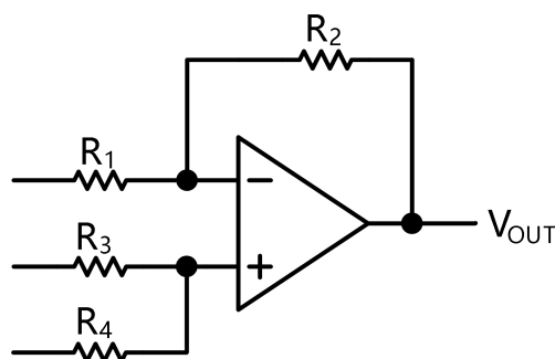
图 4. 差分放大器
