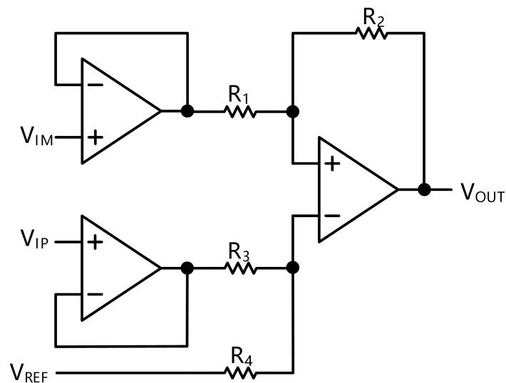
图 6. 仪表放大器
