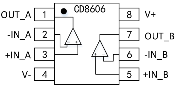
图 2.MSOP/SOP 引脚定义
