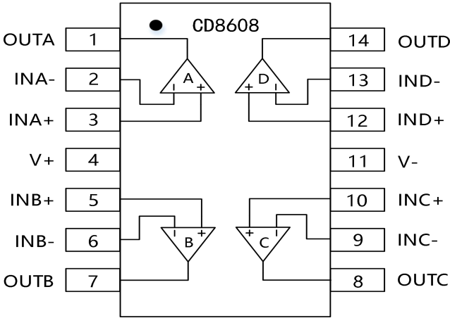
图 5.TSSOP/SOP 引脚定义
