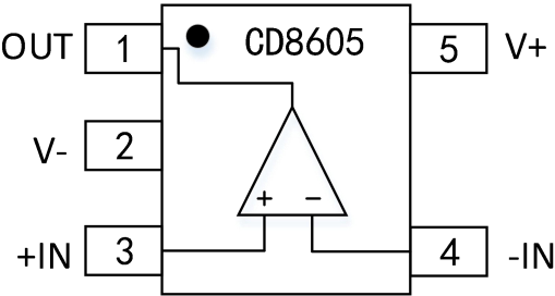
图 1.SOT23 引脚定义
