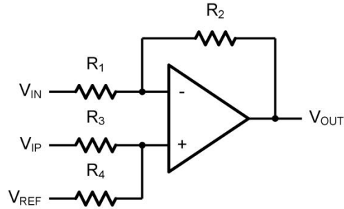
图 4. 差分放大器
