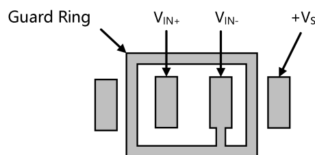
图 1. 保护环的布局
