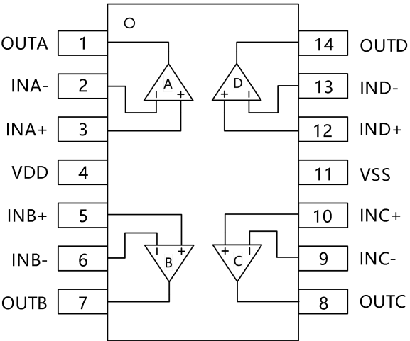
SOIC-14(SOP14), TSSOP-14
