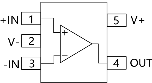
SOT23-5
