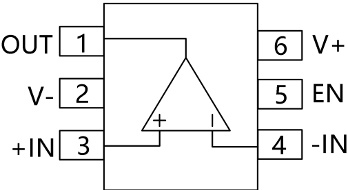
SOT23-6
