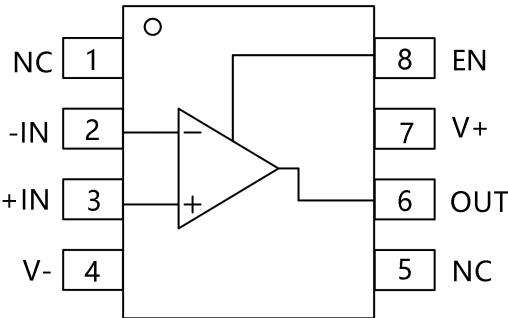
SOIC-8(SOP8)
