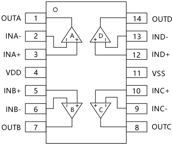
SOIC-14(SOP14),TSSOP-14
