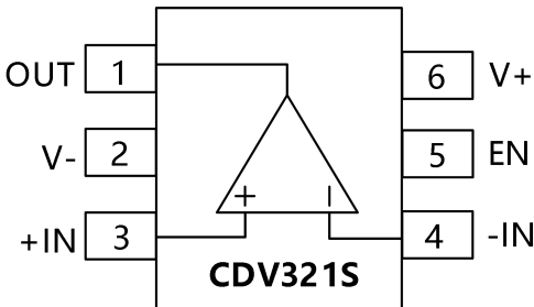
SOT23-6
