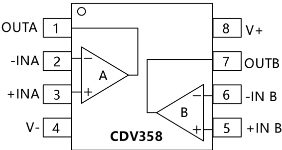
SOIC-8(SOP8),MSOP-8
