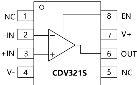
SOIC-8(SOP8)
