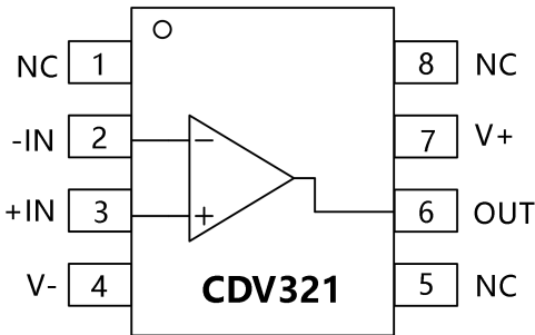
SOIC-8(SOP8),MSOP-8
