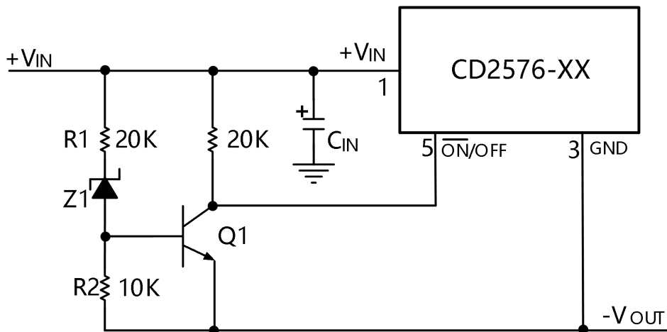
图 8 升降压电路欠压锁定
