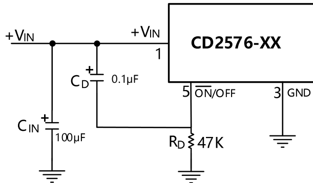
图 9. 延迟启动
