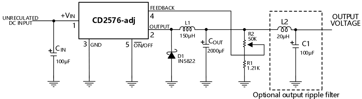
10. 低电平输出纹波电压的可调节 3A 供电电源
