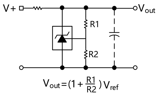
图 18. 并联电压
