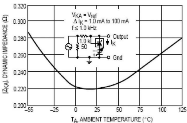
图 11.动态阻抗与环境温度关系
