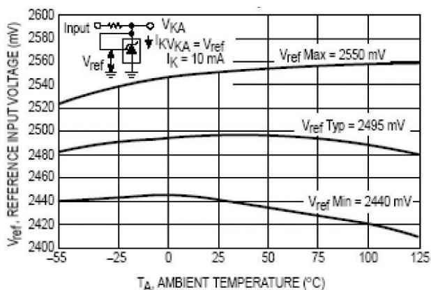
图 6. 基准输入电压与环境温度关系图
