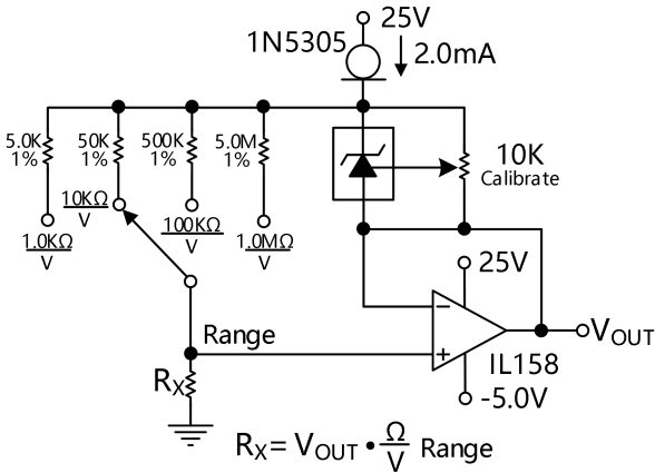
图 28. 线性欧姆计
