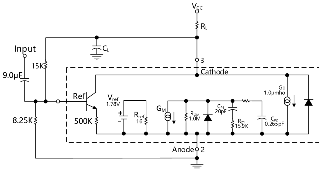
图 31.简化的 CD431 设备模型
