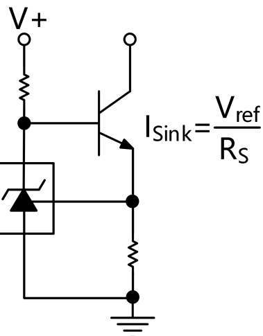
图 23. 恒定灌电流
