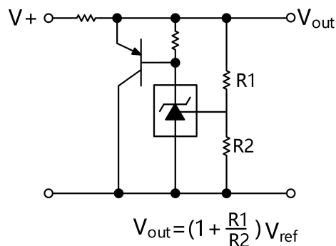
图 19. 大电流并联调节器
