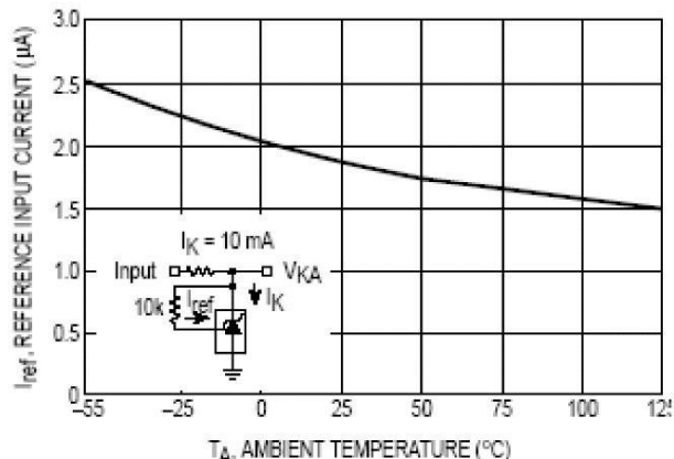
图 7. 基准输入电流与环境温度关系
