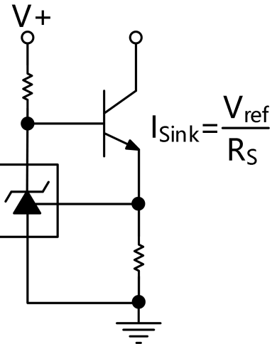
图 23. 恒定灌电流
