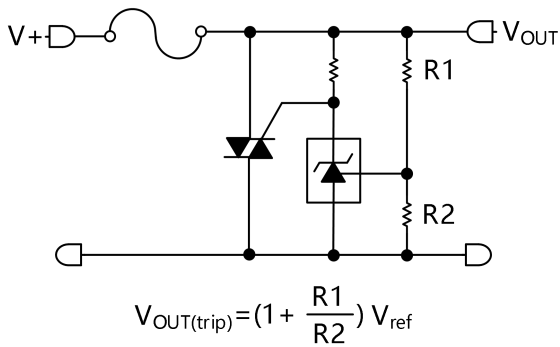
图 24. TRIAC 电路
