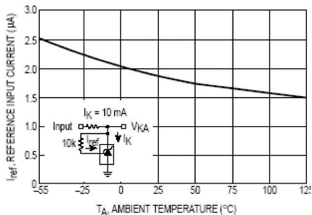
图 7. 基准输入电流与环境温度关系
