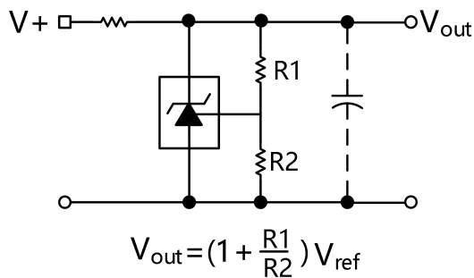
图 18. 并联电压
