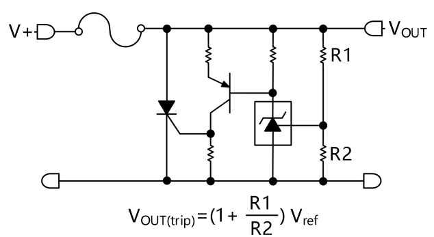
图 25. SRC 撬棍电路
