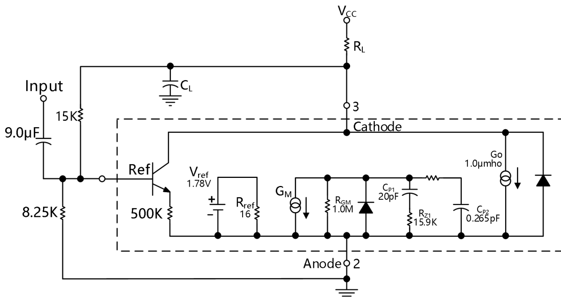
图 31.简化的 CD432 设备模型
