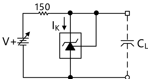
图 16. 稳定边界条件曲线 A 测试电路
