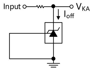
图 3. I_{off} 测试电路
