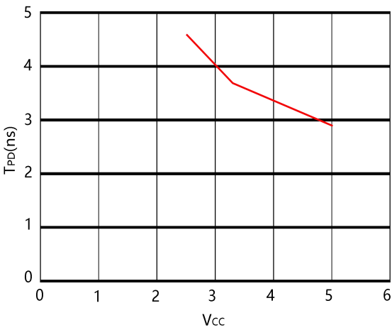
图 4. 25°C 下, T PD 和 V CC 的关系
