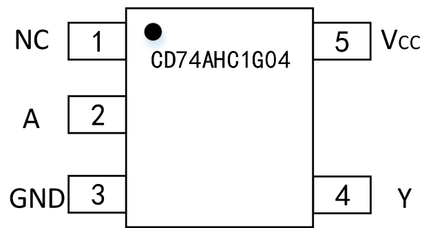
图 1. SOT23-5 引脚分配
