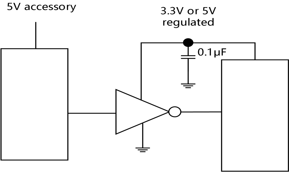
图 5 典型应用示意图
