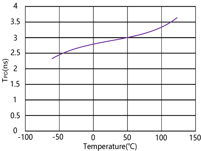
图 3. 5V 供电下, T PD 和温度的关系
