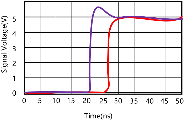
图 3.响应时间 vs 输出电压 (T A = 25°C, V A = 5 V)
