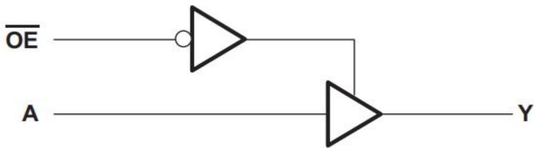
图 2. 产品框图
