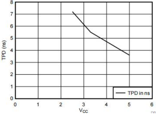
图 4.常温下, TPD 与 VCC 的关系
