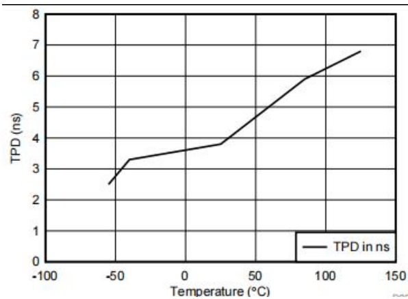
图 3.TPD 与温度的关系
