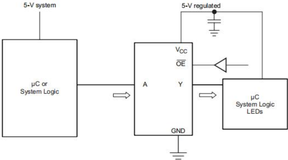
图 5 典型应用示意图
