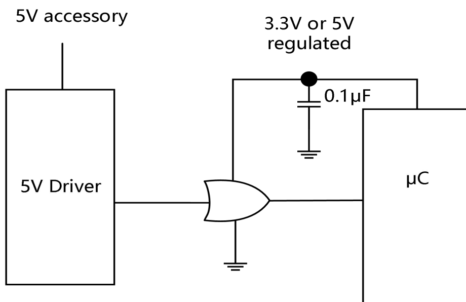
图 5 典型应用示意图
