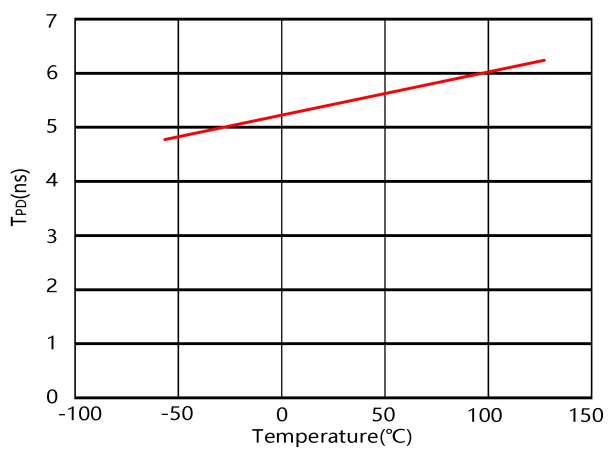
图 3. T_{PD} 和温度的关系
