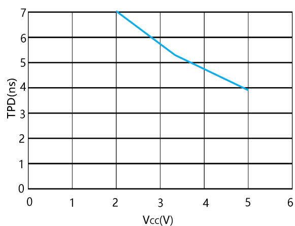
图 4. 25°C 下, T_{PD} 和 V_{CC} 的关系
