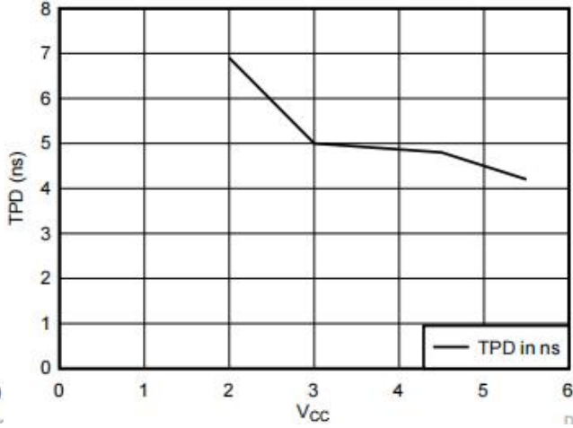
图 4. 25°C 下, T_{PD} 和 V_{CC} 的关系
