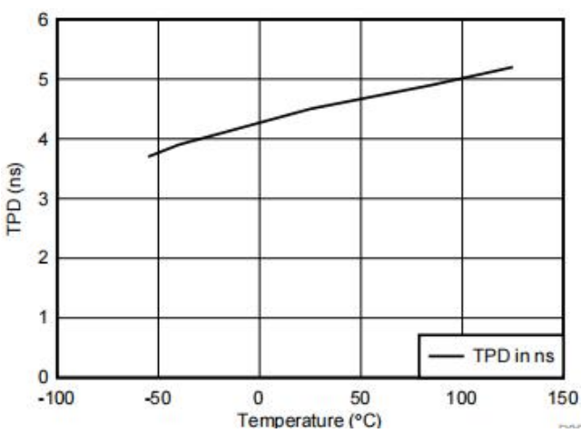
图 3. T_{PD} 和温度的关系
