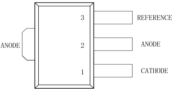
SOT89-3
