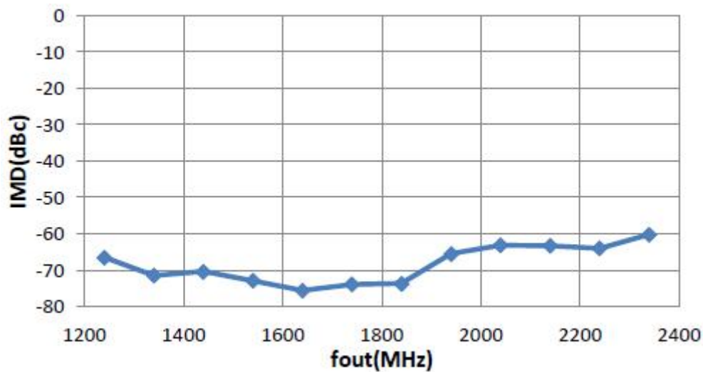
图 17 混频模式下 2.4GSPS 时 IMD 随 f_{\text{OUT}} 变化曲线
