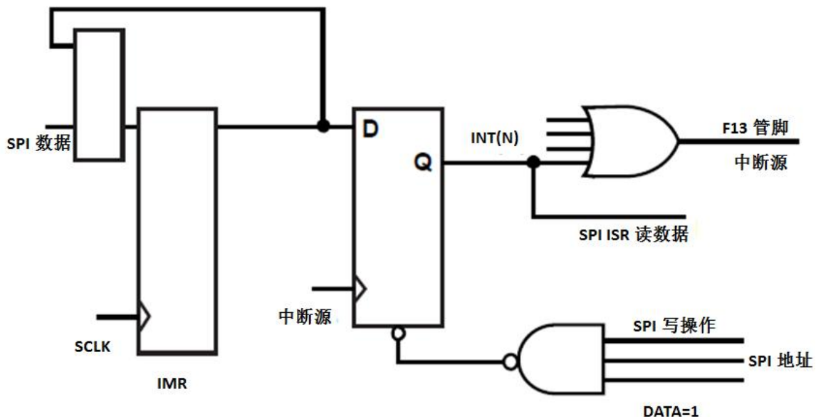
图 32 中断请求电路图
