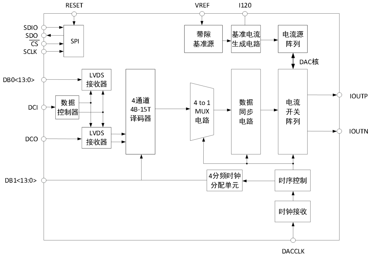
图 1. 功能框图
