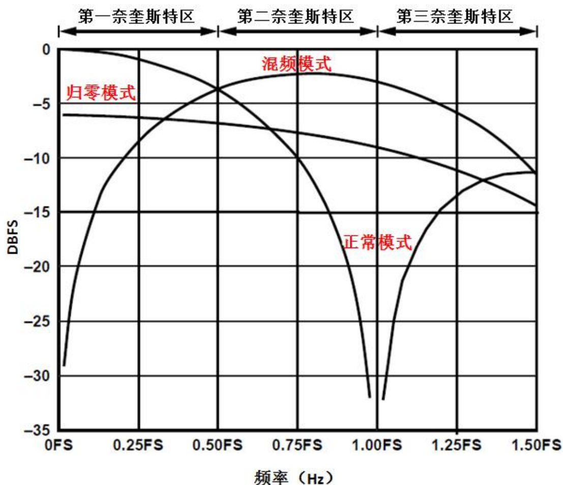
图 38 CD97D39BG 在不同模式下 SINC 函数的滚降特性
