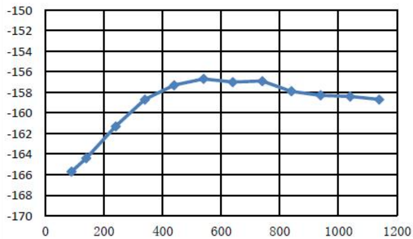
图 4 单音信号 NSD 随 f_{OUT} 变化曲线
