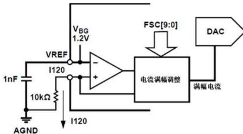
图 40 基准电压源电路
