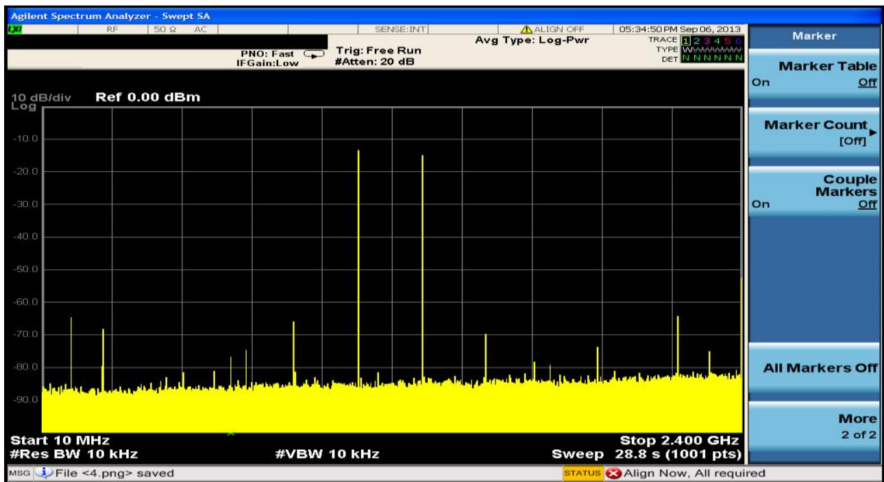
图 16 混频模式下单音信号频谱, f_{\text{OUT}}=1.31\text{GHz} , f_{\text{DAC}}=2.4\text{GSPS}
