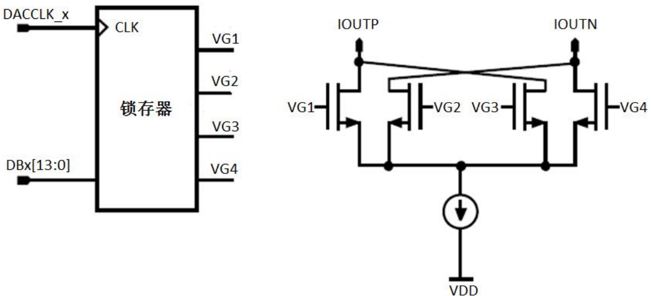
图 35 CD97D39BG 的四开关模拟输出架构
