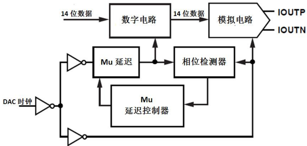
图 29 Mu 延时控制器的框图
