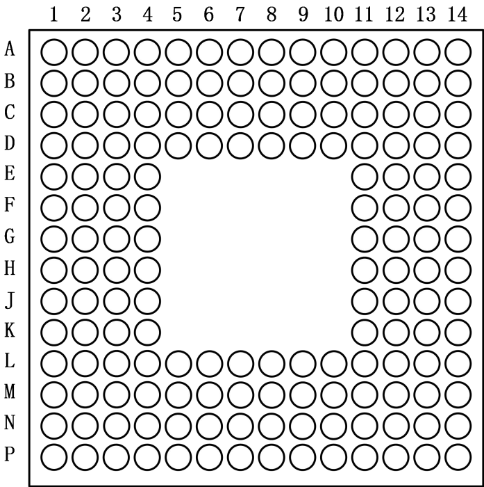
图 2. CD97D39BG 管脚图（俯视图，从器件顶部向下看的对应关系）
