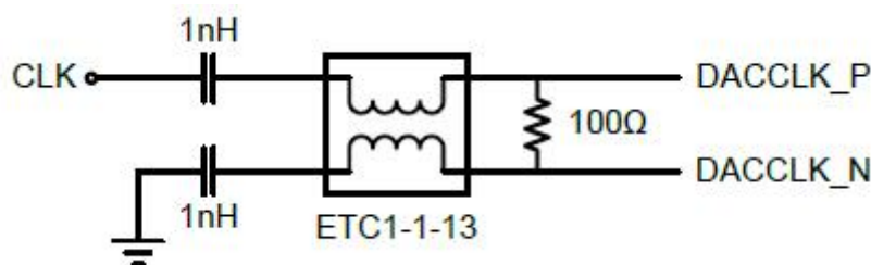
图 39 CD97D39BG 的典型时钟输入参考电路
