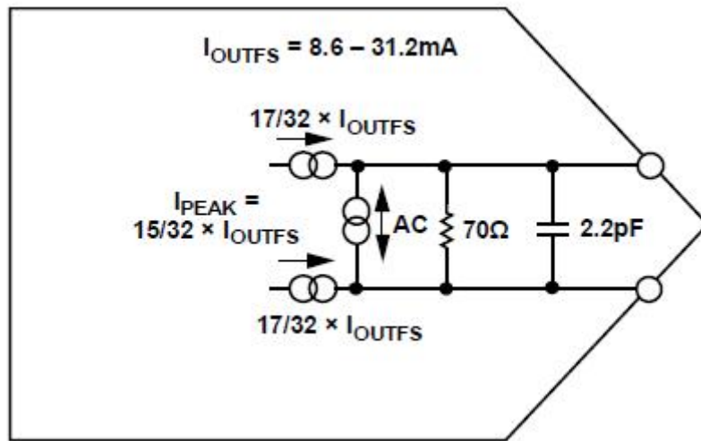
图 41 CD97D39BG 的输出等效电路
