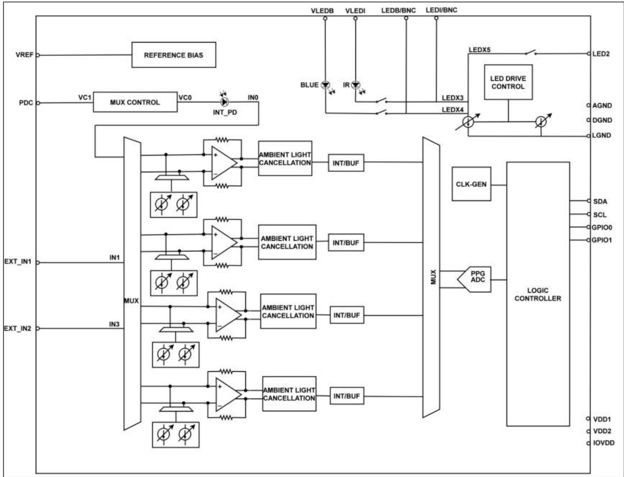
图 1.功能框图
