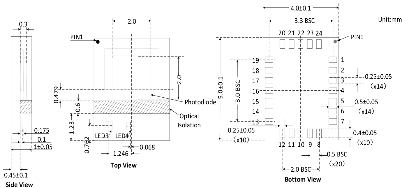
图 5 OLGA-24 尺寸图
